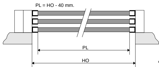
1.4. Alojamiento de Contrapesos
